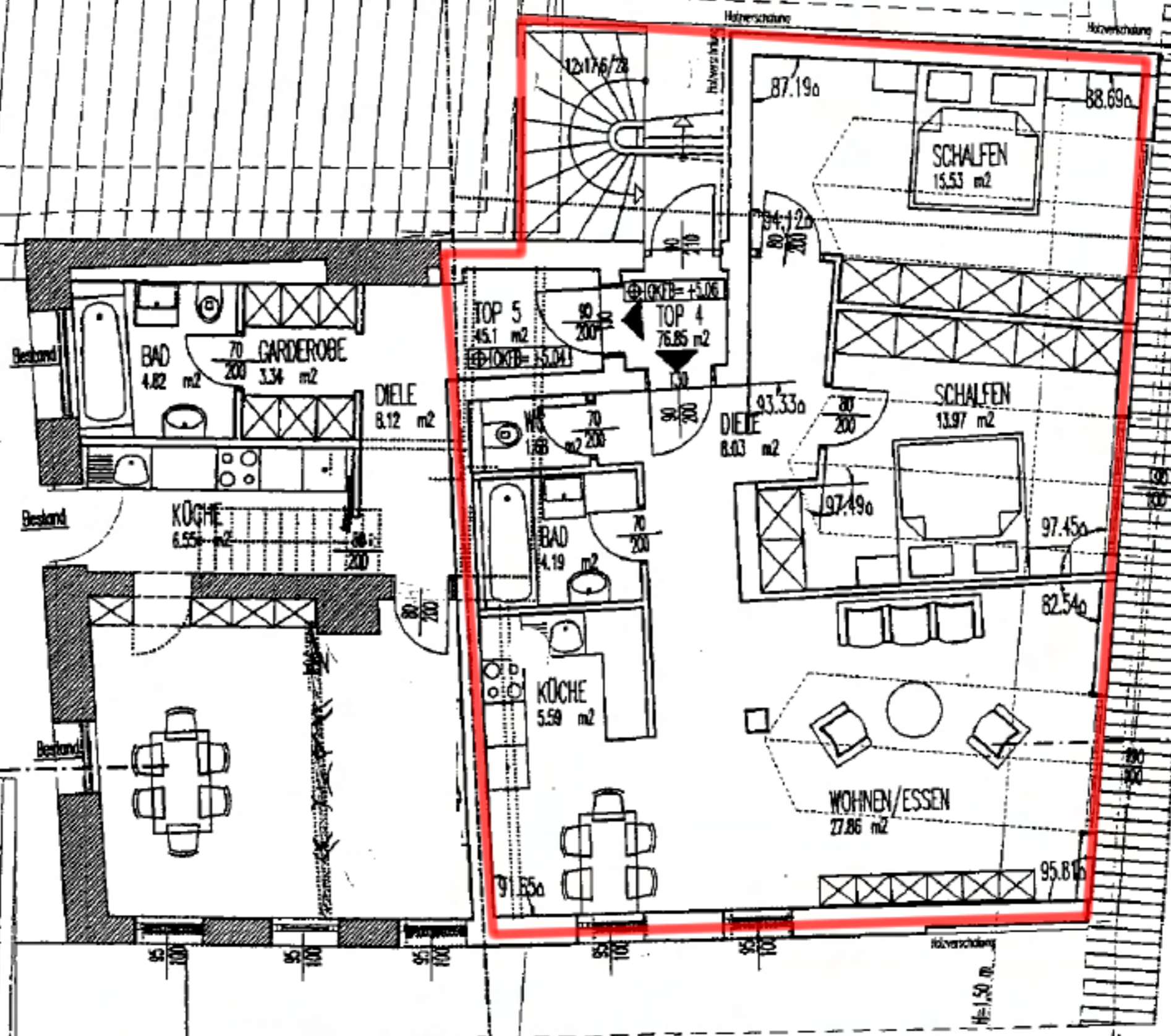
Grundriss Obergeschoss
